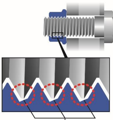
めねじに30°の傾斜を有するSpirallock®ねじ
