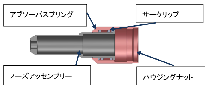
写真2 新ノーズハウジングサブアセンブリー
